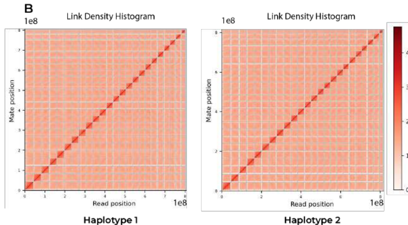
Figure B. 魚類2倍体ゲノムの ハプロタイプ分解アセンブリ のコンタクトマトリクス
